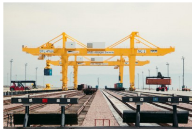
Сухой порт СЭЗ «Хоргос - Восточные ворота»
