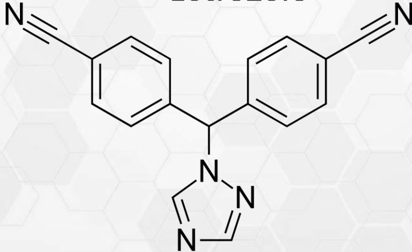
Letrozole
